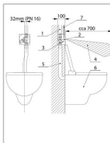
Sensor-Edelstahl-WC-Spülelektronik für Druckwasser
