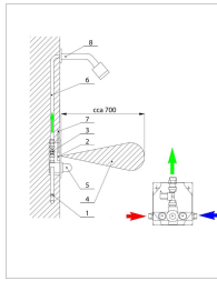
Sensor-Edelstahl-UP-Duscharmatur
