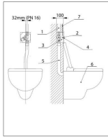
Piezo-Edelstahl-WC-Spülelektronik für Druckwasser
